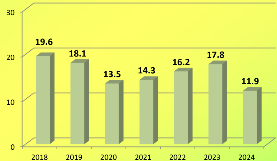
■ Картофель, тыс.тонн
