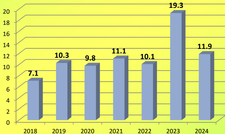
■ Подсолнечник, тыс.тонн
