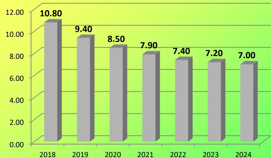
■ Овощи, тыс.тонн
