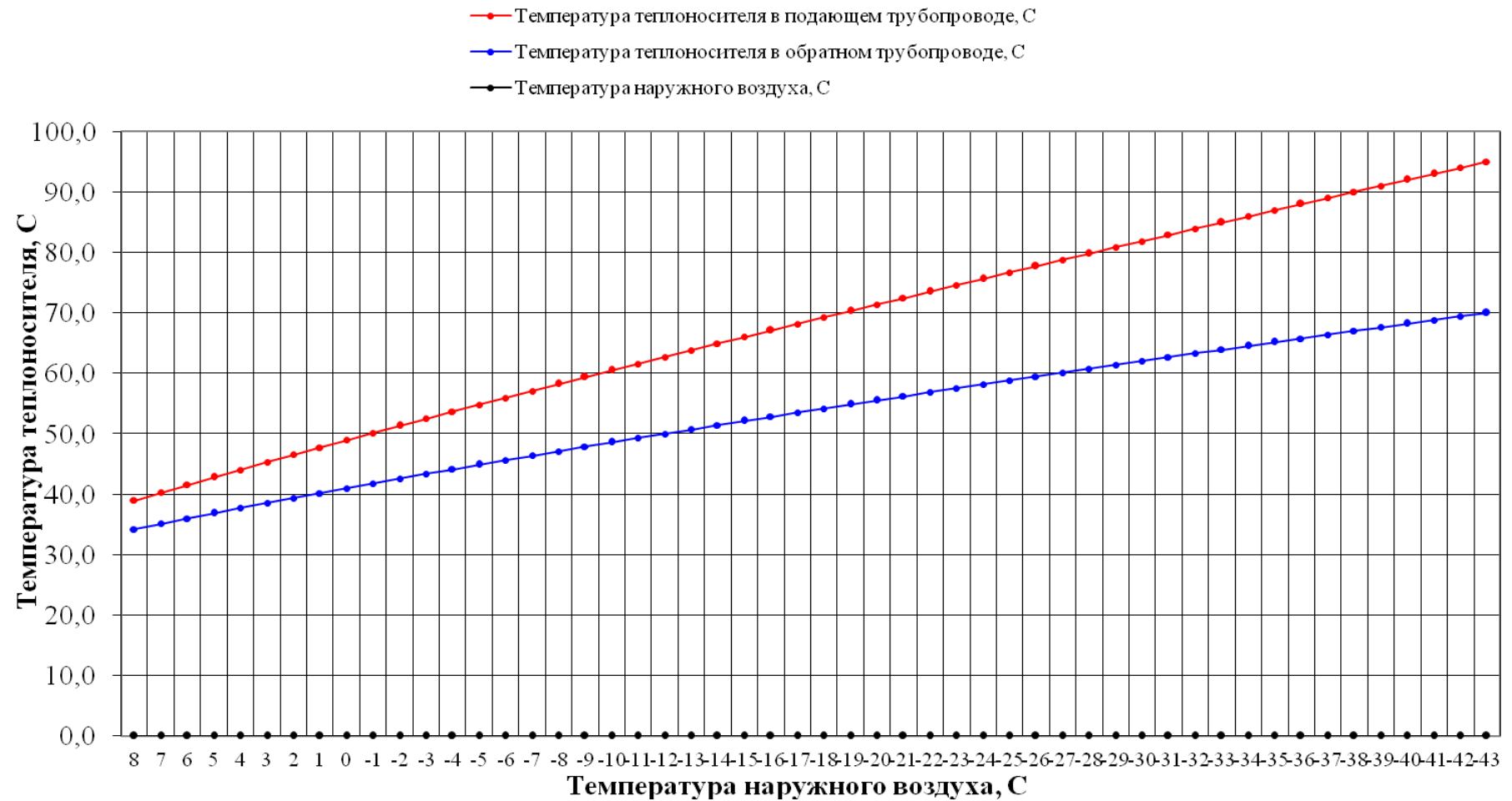
Рис.1 Температурный график работы котельных с.Чемодановка
